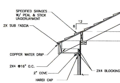
2 A.5 DETAIL SCALE: N.T.S.
