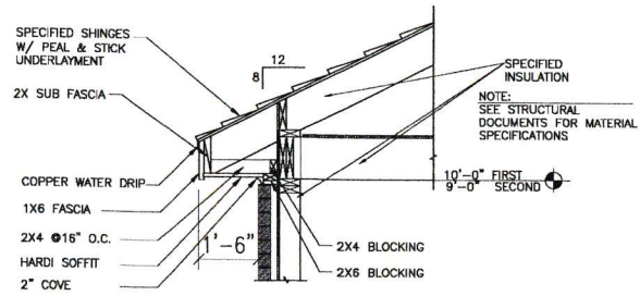
1 A.5 DETAIL SCALE: N.T.S.
